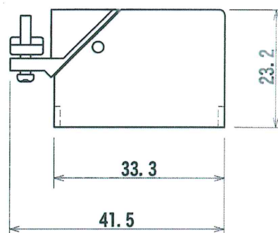
20芯【SL】CV-020-SL 横出しカバー（太線用）
