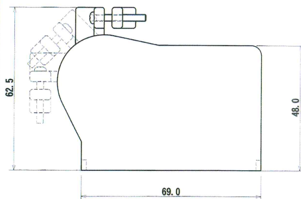
120芯【SP45】 CV-120-SP45 分割式縦横45度兼用カバー
