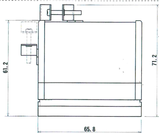
90芯【DV】 CV-090-DV 分割45度カバー
