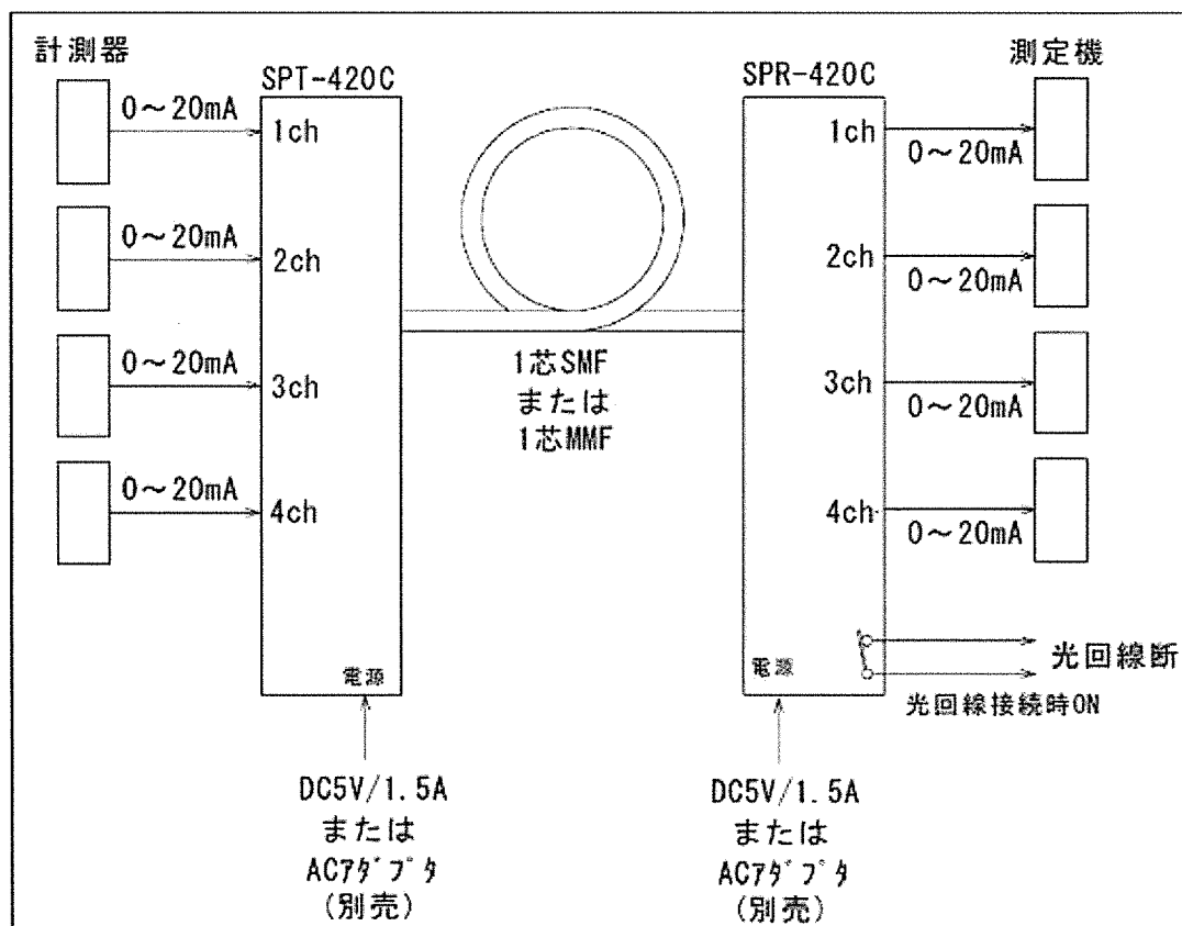
図1 接続構成
