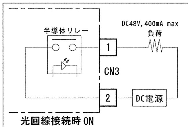
出力構成
