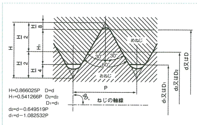
● メートル並目ネジ(JIS B 0205)寸法表
