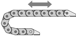
(a). 水平スライド取付け① (上面スライド)
