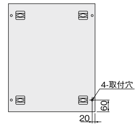
■キャビネット取付穴推奨寸法 (取付穴はあいていません。)
